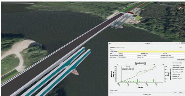
Abbildung 4: Bauablaufssimulation mit Baufortschrittsanzeige zum Pilotprojekt Petersdorfer Brücke (Quelle: DEGES)
